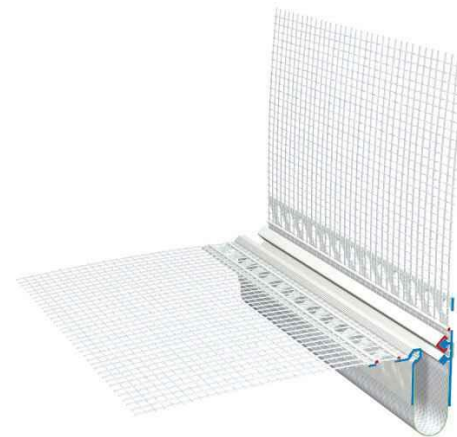
Dehnfugenprofil Typ V für versetzte Wandflächen
